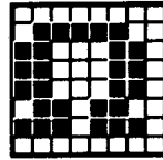
191 &HBF &X101111111
