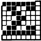
190 &HBE &X101111110
