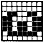
189 &HBD &X101111101
