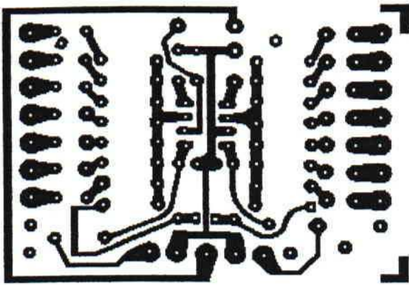
Fig. 2 Le circuit imprimé
